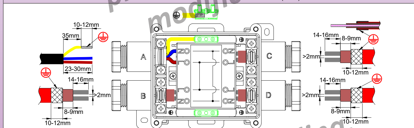
Modèle à 3 câbles chauffants et un câble d'alimentation (YB14)
