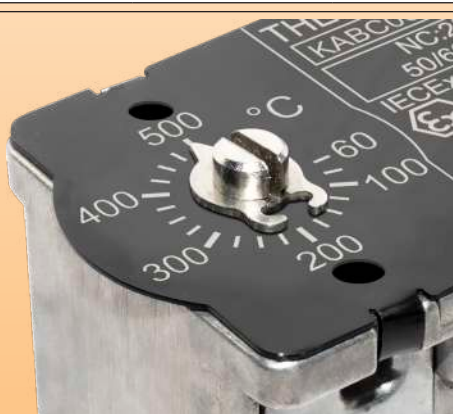
C : Réglage par tournevis et clips flèche, sur cadran aluminium imprimé, pour utilisation dans les boîtiers EX-e en PPS de JPCI ou d'autres fournisseurs en traçage électrique ;
