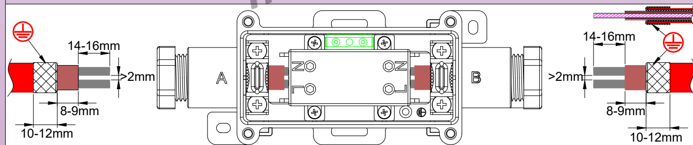
Modèle à deux câbles chauffants (YB02)
