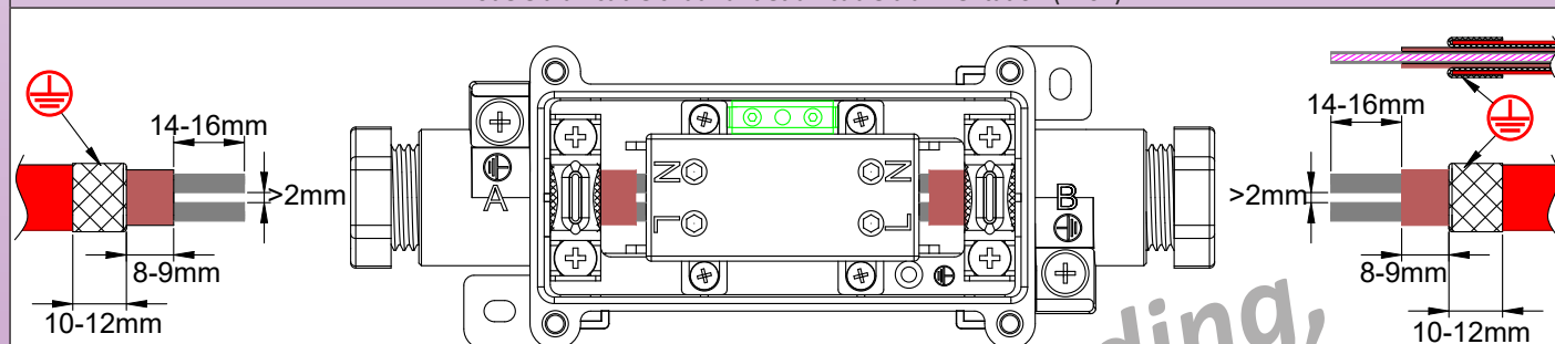
Modèle à un câble chauffant et un câble d'alimentation (Y401)
